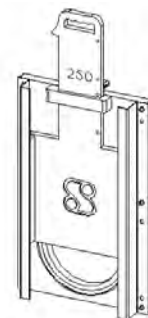
Vatech HDPE håndspjæld. For vægmontage. Vatech nr. 228001.0xx
