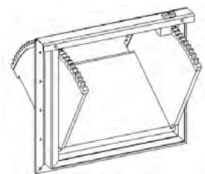
Vatech HDPE overløbsvugge. Materialer: HDPE/AISI 316. Vatech nr. 228009.0xx
