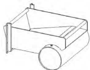
Vatech HDPE overløbsunit med flyder. Materialer: HDPE/AISI 316. Vatech nr. 228010.5xx
