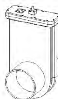
Vatech HDPE skydeventil med PE-ender. Hus og spjældplade af HDPE. Spindel af syrefast stål AISI 316. Vatech nr. 410570.0xx
