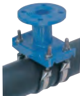
Universal anboringsbøjle. Med flangefang. Pris uden bagbøjler. Vatech nr. 101492.0xx
