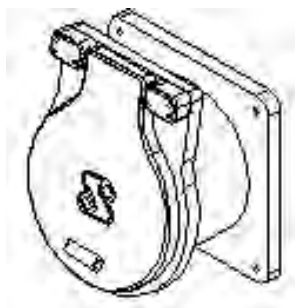
Vatech HDPE udløbsklap. Afvinkling 10°. Tilslutning: Vægflange. Type TKV-A. Vatech nr. 226000.1xx
