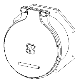
Vatech HDPE udløbsklap. Afvinkling 10°. Tilslutning: Vægflange. Type TKV-A. Vatech nr. 226000.3xx
