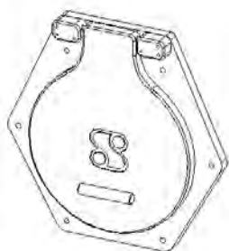
Vatech HDPE udløbsklap. Tilslutning: Vægflange. Type TKV. Vatech nr. 226001.2xx
