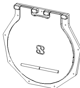
Vatech HDPE udløbsklap. Tilslutning: Vægflange. Type TKV. Vatech nr. 226001.3xx
