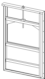
Vatech HDPE overløbsspjæld. For vægmontage. Med 1 spindel. Vatech nr. 228005.0xx
