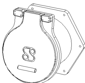
Vatech HDPE udløbsklap. Afvinkling 10°. Tilslutning: Vægflange. Type TKV-A. Vatech nr. 226000.2xx
