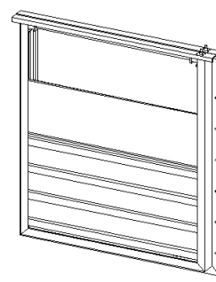
Vatech HDPE overløbsspjæld. Dobbelt spjældplade. 2 spindler pr. spjældplade. For vægmontage. Vatech nr. 228007.0xx
