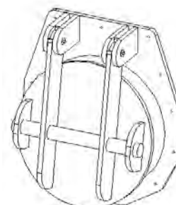
Vatech HDPE udløbsklap. Afvinkling 10°. Tilslutning: Vægflange. Type TKV-A. Vatech nr. 226000.4xx
