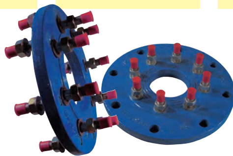
Stbj. flangereduktion. Epoxybehandlet. PN 10. Vatech nr. 131166.xxx
