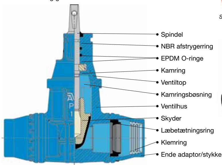
Serie 16/29 - Med trækfast indstiksmuffe til PE-rør / udvendigt konisk rørgvind
