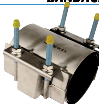
Rustfri bandagemuffe. Dobbeltrækket. Vatech nr. 101320.0xx
