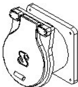
Vatech HDPE udløbsklap. Afvinkling 10°. Tilslutning: Vægflange. Type TKV-A. Vatech nr. 226000.1xx
