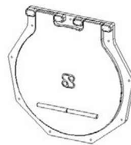
Vatech HDPE udløbsklap. Tilslutning: Vægflange. Type TKV. Vatech nr. 226001.4xx
