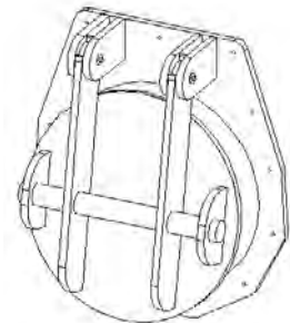
Vatech HDPE udløbsklap. Afvinkling 10°. Tilslutning: Vægflange. Type TKV-A. Vatech nr. 226000.4xx
