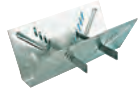
Vatech galvaniseret forankringsplade for stikledningsventiler. Vatech nr. 145281.012
