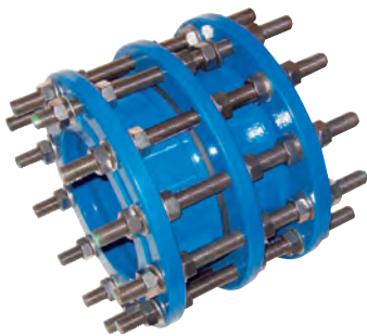
Vatech ekspansionsstykke. Epoxybehandlet stål. Andre materialer på forespørgsel. Forskydelig 25 mm. Vatech nr. 141900.xxx
