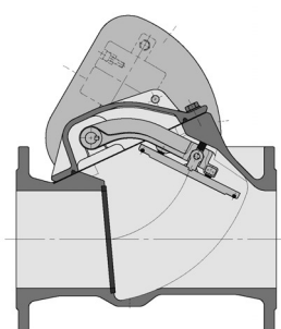
ERHARD kontraklapventil med afskærmning for arm og lod.
